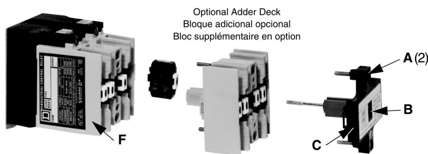
FIG. 1 : AC Control Relay: TYPE X, Series A / Relevador de control de ~ (c.a.): TYPE X, serie A / Relais de contrôle ca : TYPE X, série A
