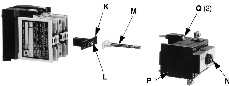
FIG. 3 : Latch Attachments / Aditamentos de bloqueo / Accessoires de verrouillage
