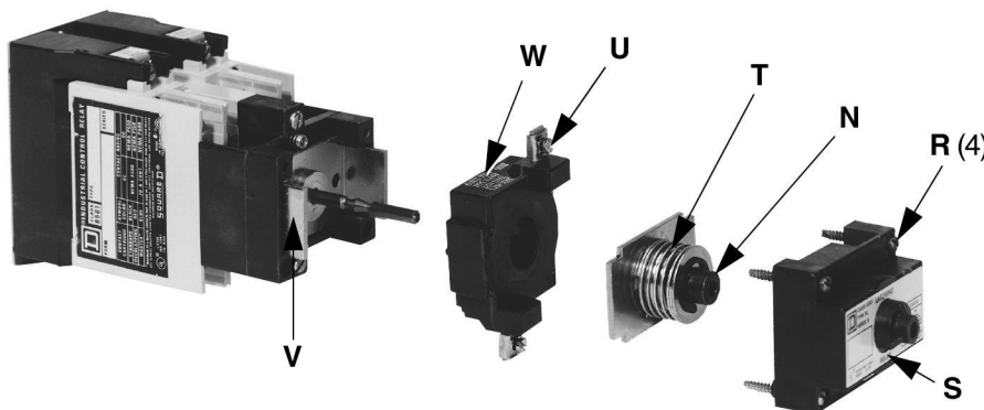
FIG. 5 : Unlatch Coil Replacement / Reemplazo de la bobina de desenganche / Remplacement de la bobine de déverrouillage
